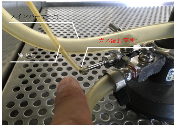
種火用シリコンチューブの亀裂
