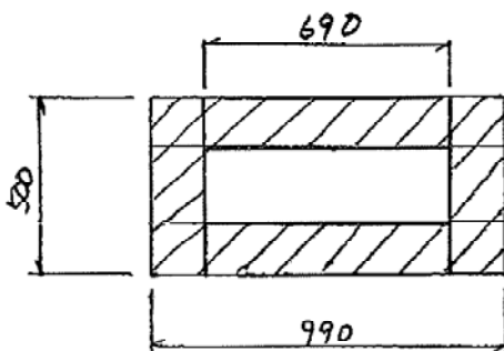
篩を載せる架台の寸法（単位：mm）
